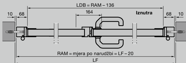
2-krilna bočna vrata s aluminijskim blok okvirom tip profila 2 Ugradnja iza otvora
