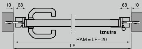
Bočna vrata s aluminijskim blok okvirom, profil tipa 2 Ugradnja iza otvora
