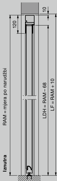
Bočna vrata s aluminijskim blok okvirom, profil tipa 2 Ugradnja iza otvora
