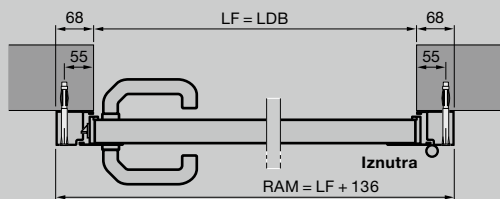
Bočna vrata s aluminijskim blok okvirom, profil tipa 1 Ugradnja iza otvora
