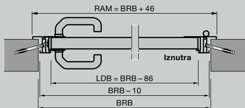
Bočna vrata s aluminijskim kutnim okvirom, profil tipa 3 Vanjski nosač
