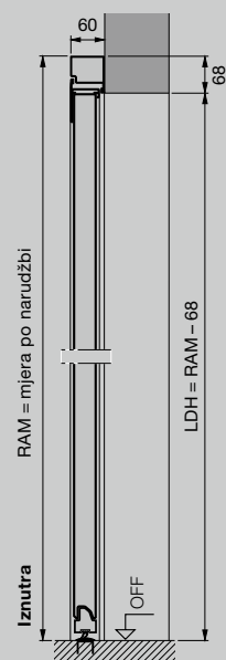
Bočna vrata s aluminijskim blok okvirom, profil tipa 2 Ugradnja iza otvora
